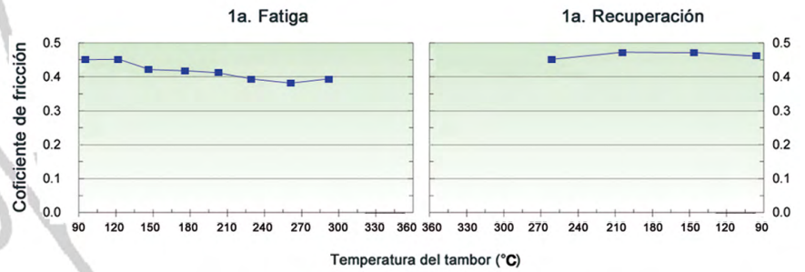
GRÁFICAS DE FATIGA Y RECUPERACIÓN Y DESGASTE
